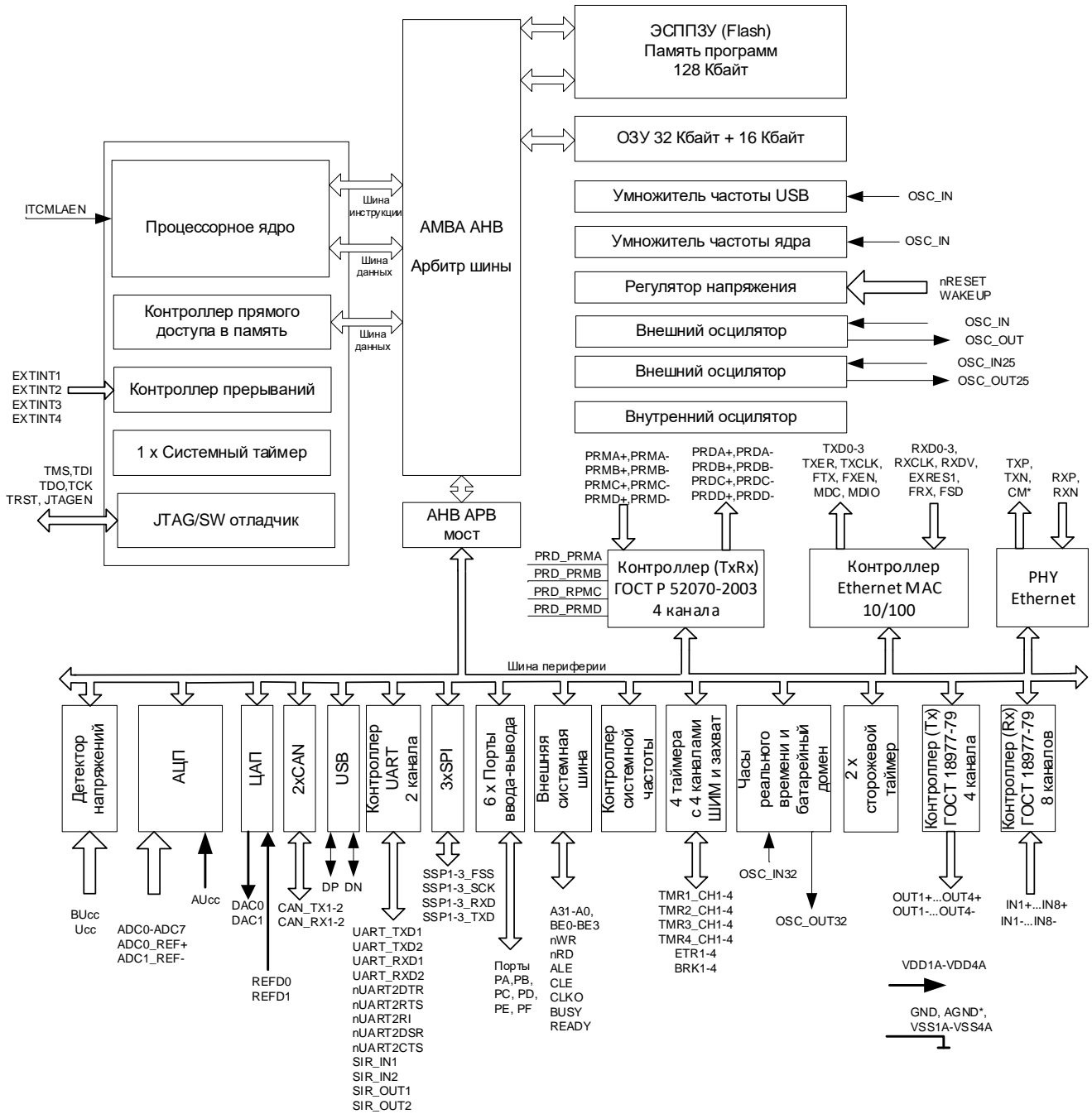
Рисунок 1 – Структурная блок-схема
