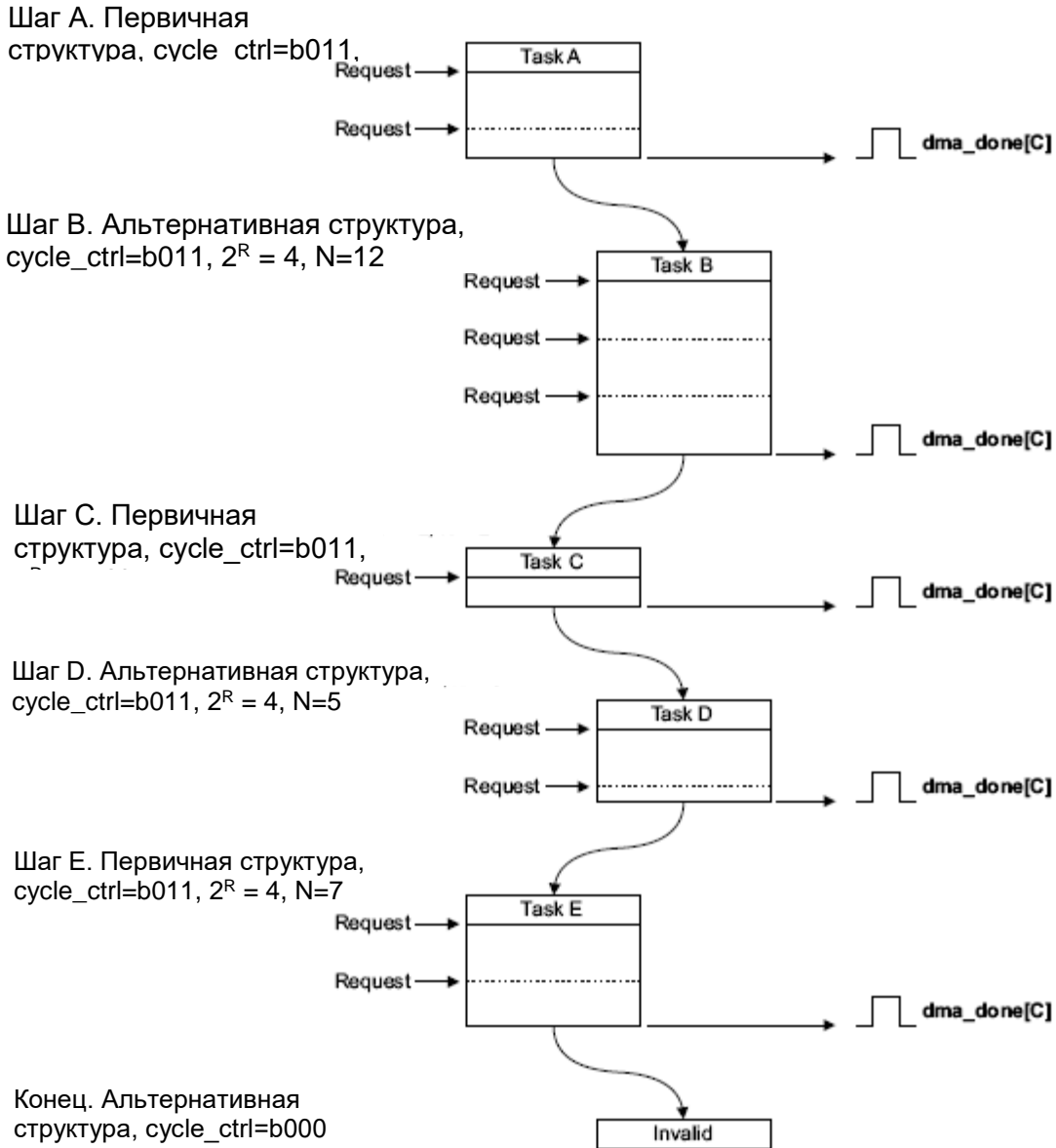
Рисунок 126 – Пример функционирования контроллера в режиме «пинг-понг»
