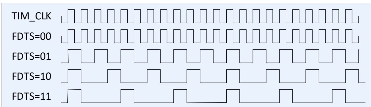
Рисунок 67 – Диаграмма тактовой частоты F_{DTS} в зависимости от значения FDTS[1:0] в регистре CNTRL
