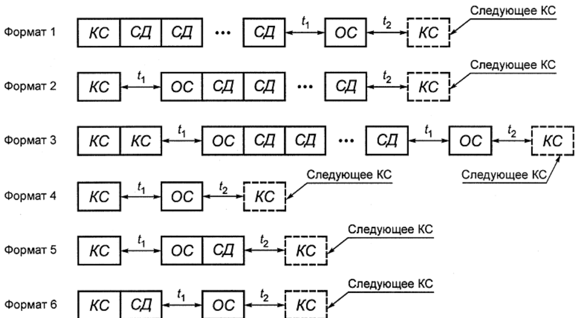
Рисунок 55 – Форматы сообщений
