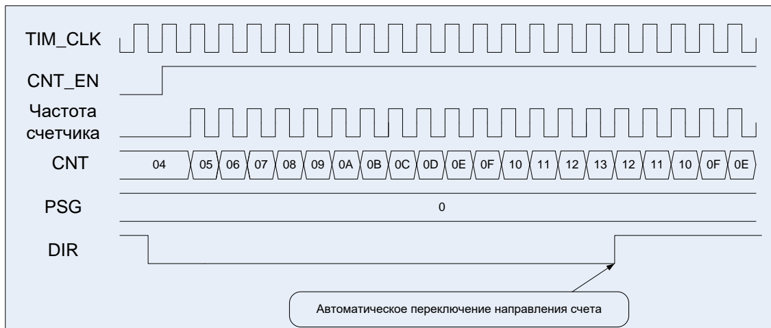
Рисунок 64 – Диаграммы работы таймера, счет двунаправленный, сначала прямой
