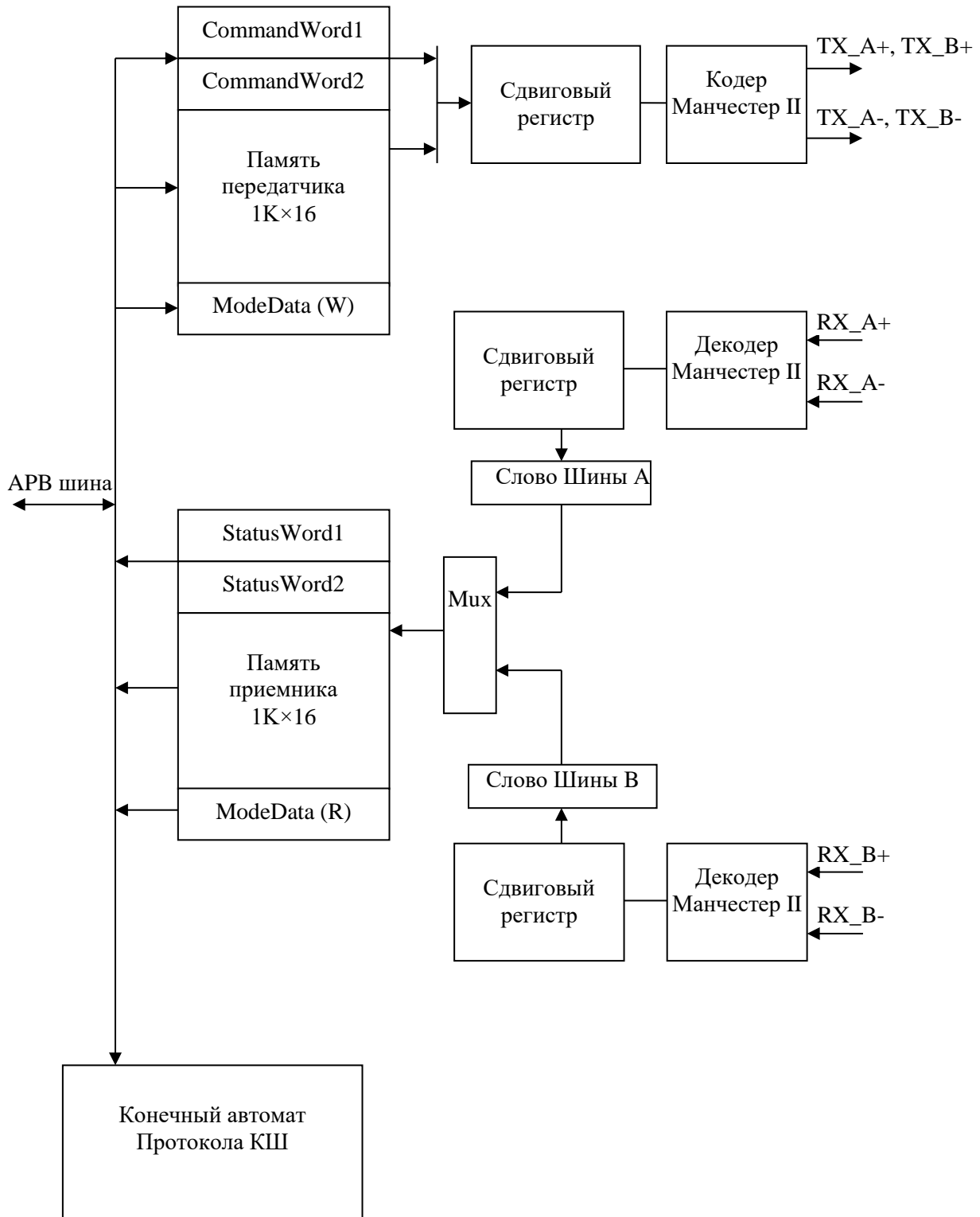
Рисунок 58 – Структурная схема работы в режиме КШ
